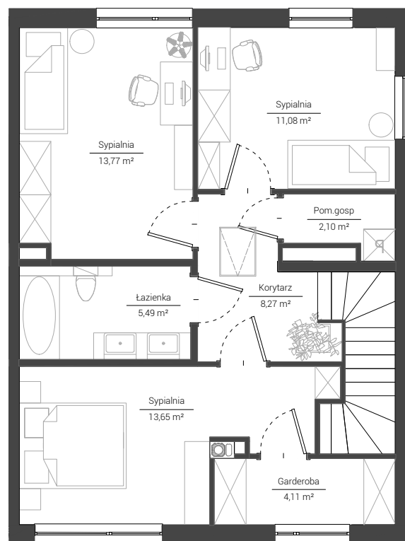
PIĘTRO
